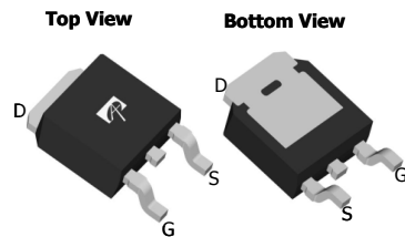
TO252 DPAK
