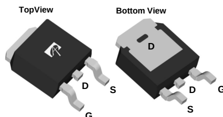
TO252 DPAK: AOD516
