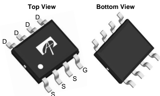
SOIC-8
